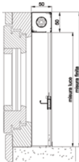
Sez. verticale
