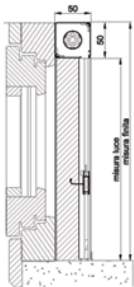
Sez. verticale
