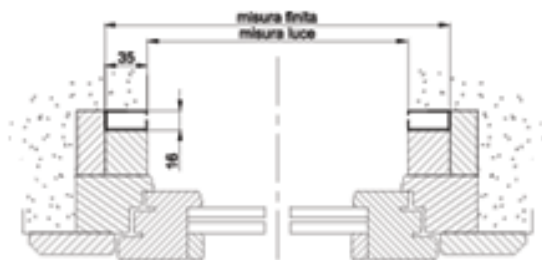
Sez. orizzontale
